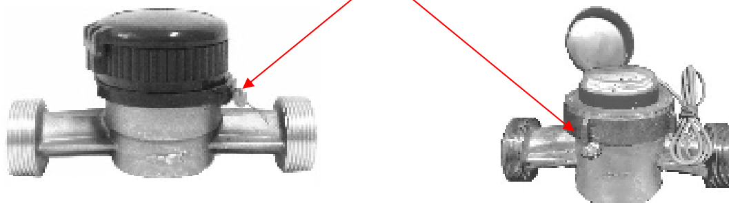
Рисунок 5 - Схема пломбировки счетчиков модификаций ОСВХ и ОСВУ
