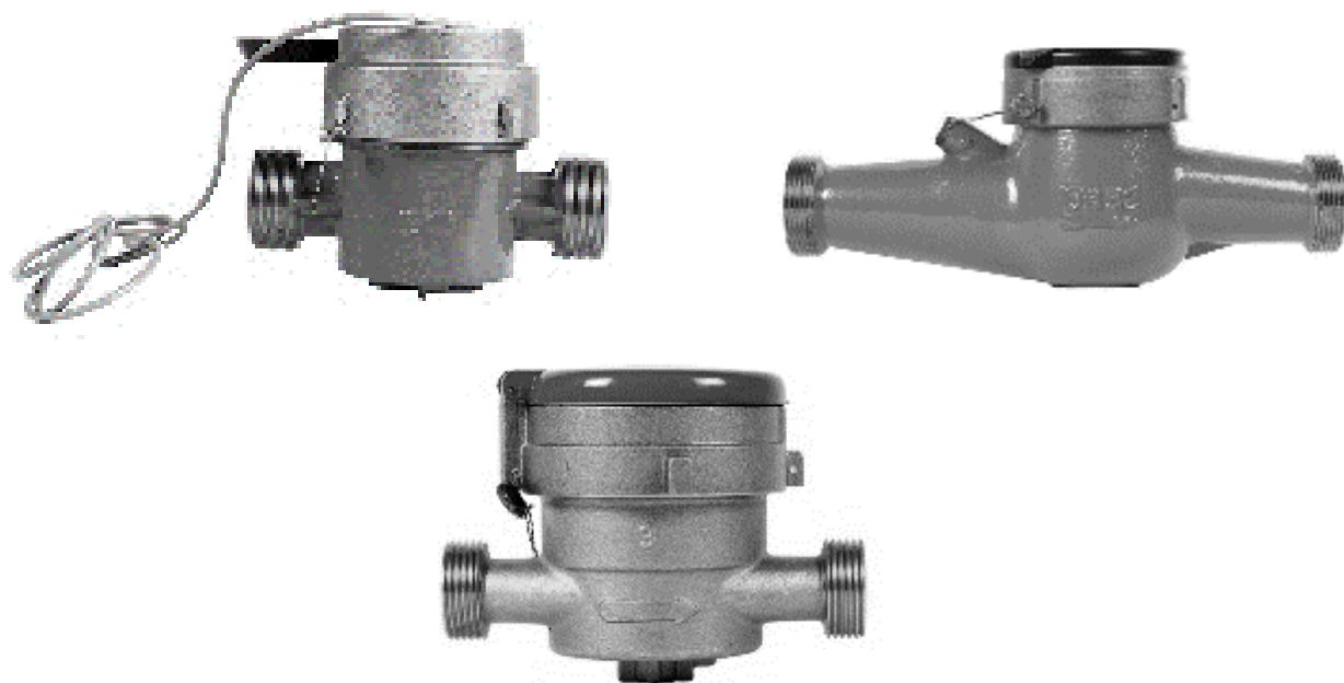
Рисунок 3 - Общий вид счетчиков модификаций VKM и VKM M
