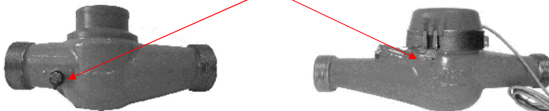
Рисунок 6 – Схема пломбировки счетчиков модификаций ВСКМ 90 и ВСКМ 90Х
