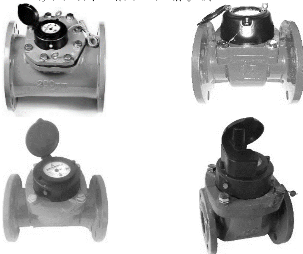
Рисунок 3 - Общий вид счетчиков модификаций VKM и VKM M
